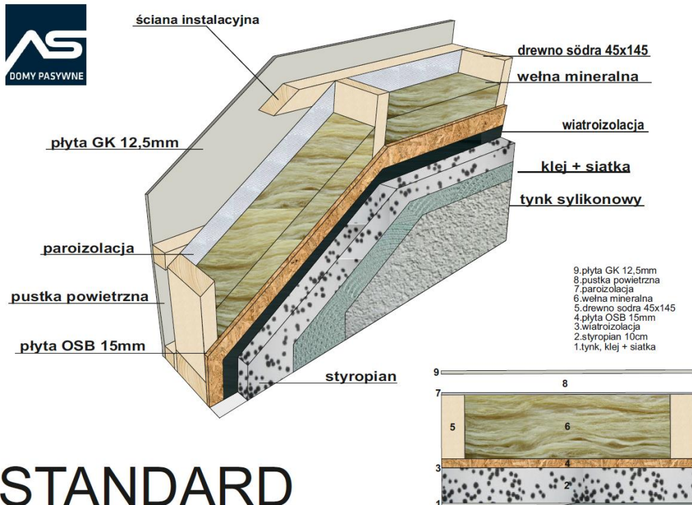
Rys. 2 Przekrój ściany zewnętrznej.
